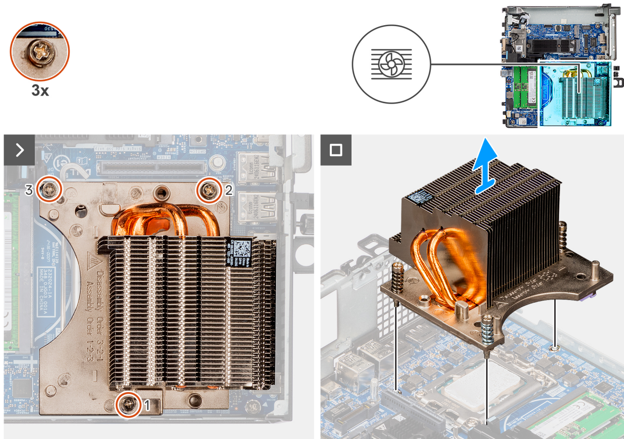
Abbildung 46. Kühlkörper entfernen
