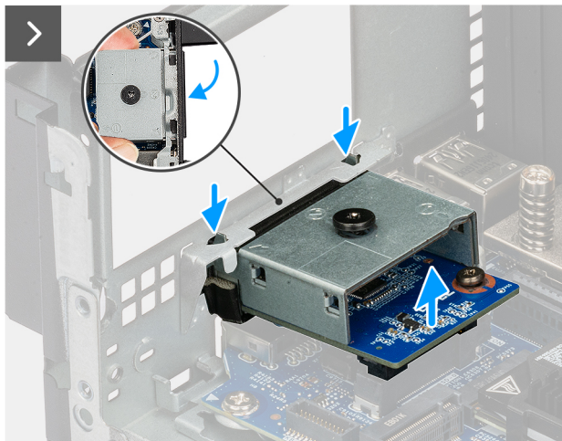
Abbildung 45. Entfernen des HDMI-Anschlusses
