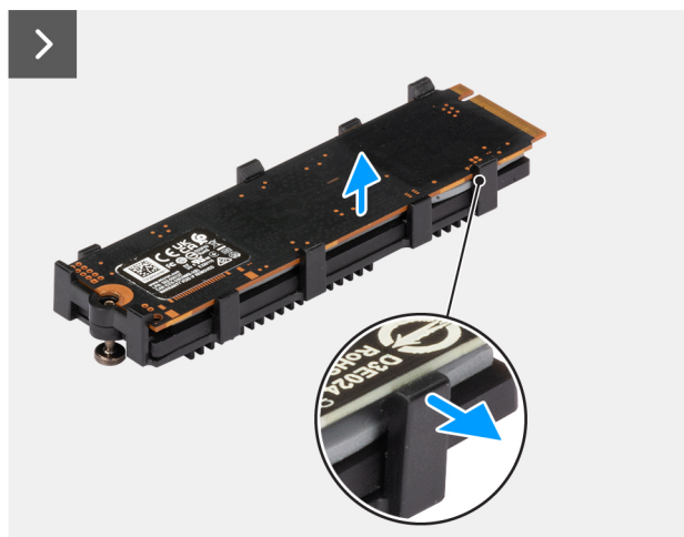
Abbildung 21. Entfernen des M.2-2280-PCIe-Solid-State-Laufwerks (Steckplatz 1)
