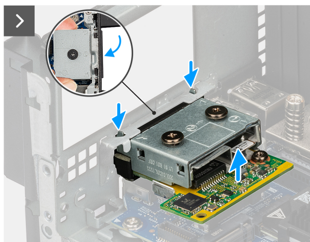
Abbildung 33. Entfernen des optischen 5G-Glasfaseranschlusses
