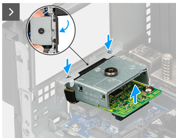
Abbildung 39. Entfernen des DisplayPorts
