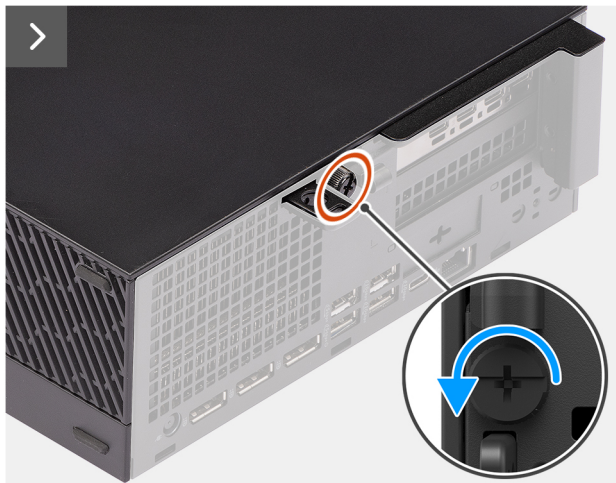
Abbildung 3. Entfernen der Seitenabdeckung
