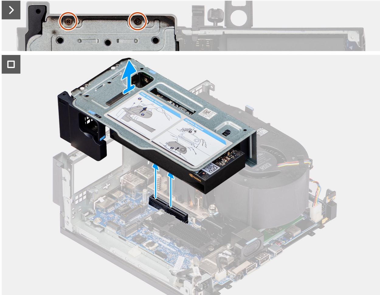
Abbildung 9. Entfernen des Riser-Kartenmoduls
