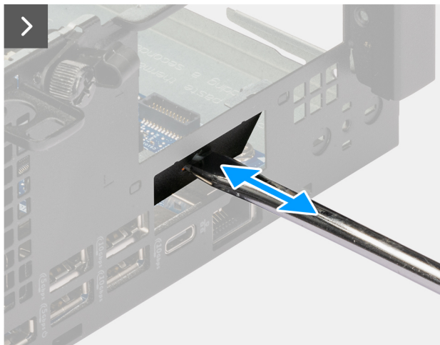
Abbildung 43. Einbauen des HDMI-Ports
